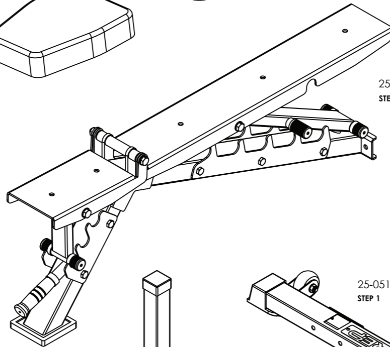
25-0824 STEP 1 x1
